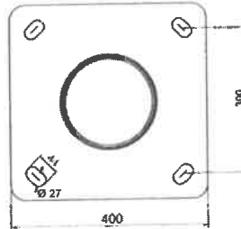
10-12 MÉTERES OSZLOPOKHOZ
