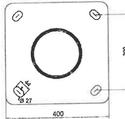
10-12 MÉTERES OSZLOPOKHOZ
