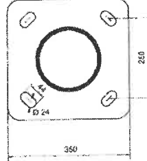
6-9 MÉTERES OSZLOPOKHOZ
