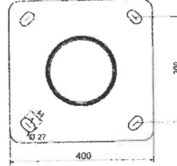
10-12 MÉTERES OSZLOPOKHOZ
